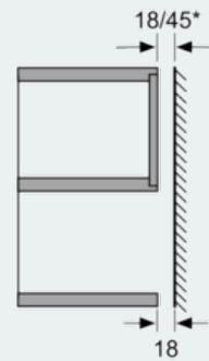
* = Valor para aparelhos com grill Medidas em mm
